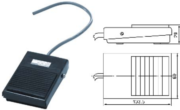
LLJFS1-1(铁壳Iron cover)
